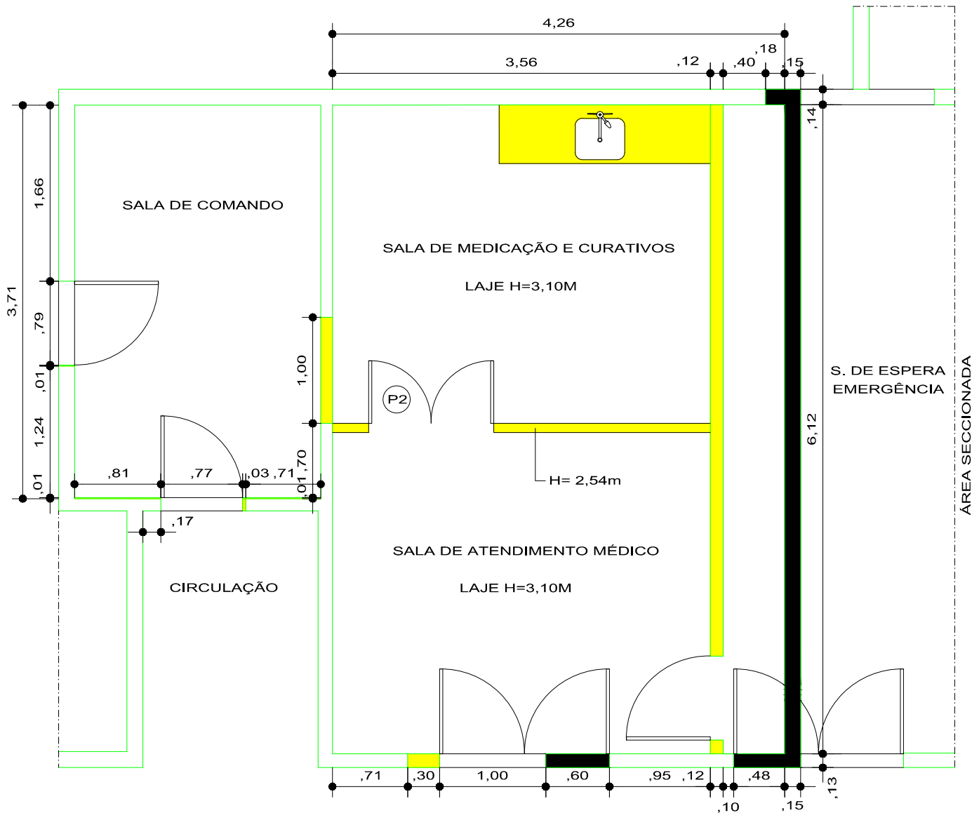
PLANTA-BAIXA DE REFORMA ESCALA=1/50
