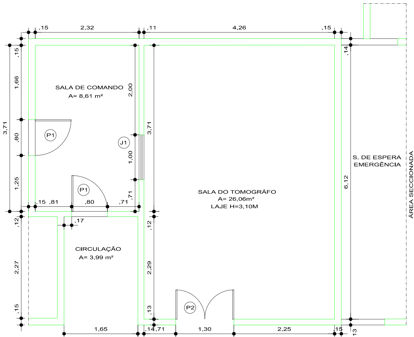
PLANTA-BAIXA PÓS-REFORMA ESCALA=1/50
