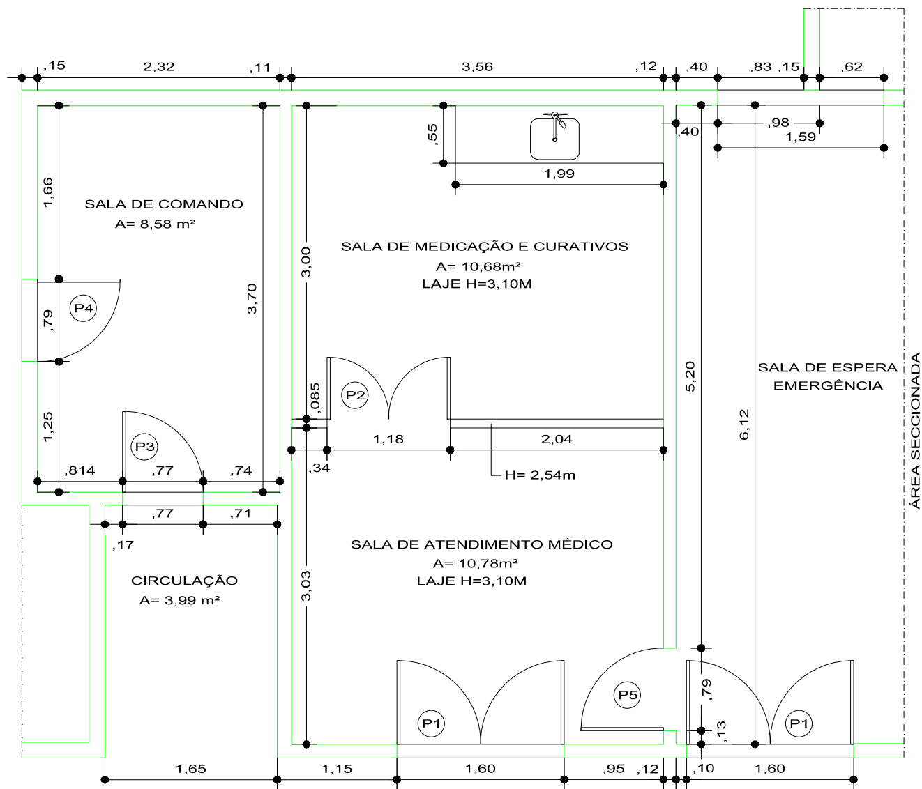
PLANTA-BAIXA TÉCNICA ATUAL ESCALA=1/50
